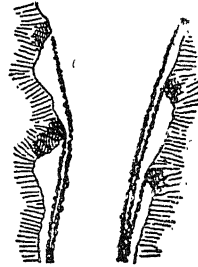
चित्र १८१—पार्श्व मोरेन्स।
